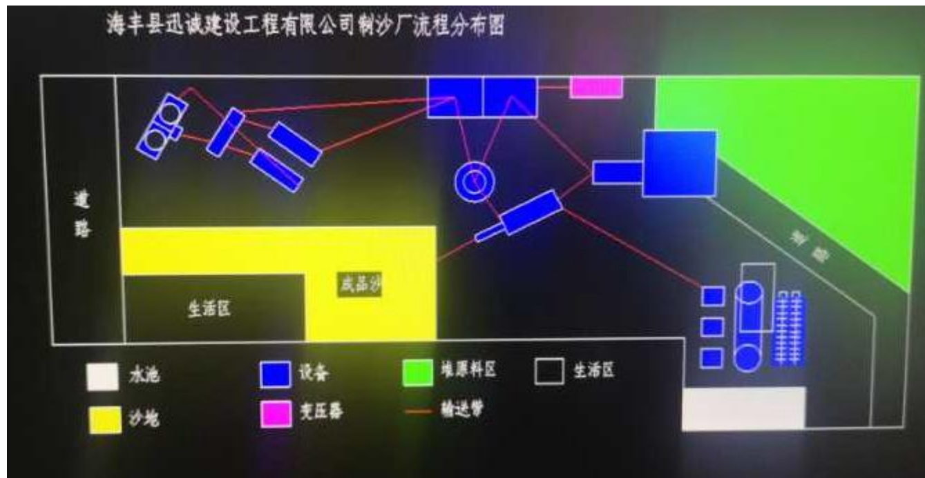
附图6 项目平面布置图
