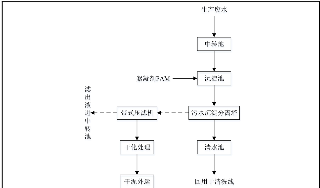
图 7-1 项目洗砂废水处理工艺流程图
