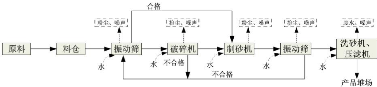
图 5-2 项目生产工艺流程图
